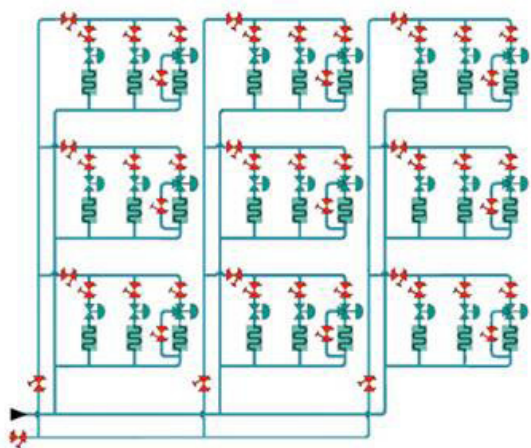
Статические балансировочные клапаны
