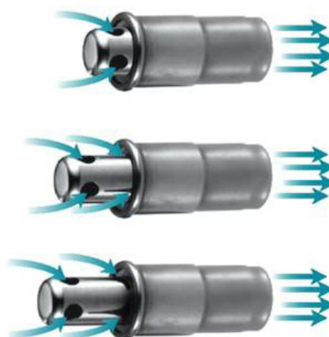
Работа картриджа SS, при изменении давления
