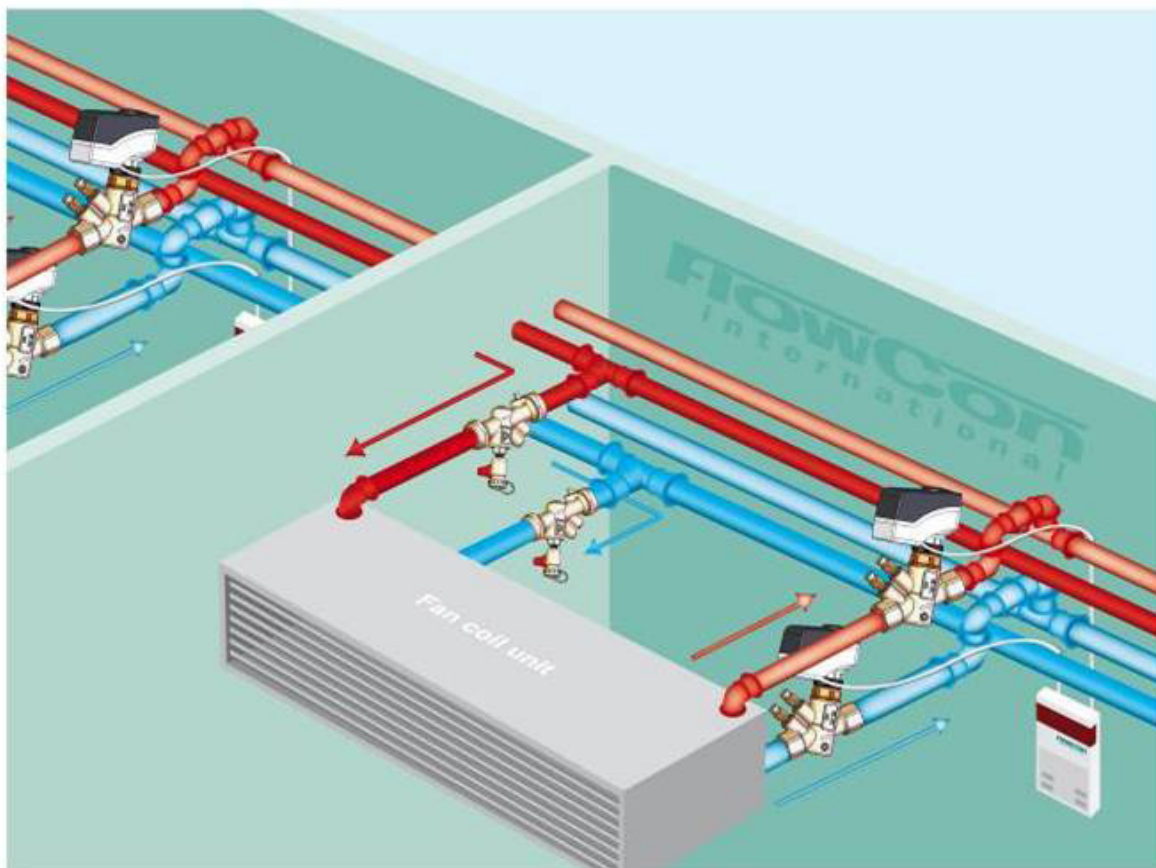
Система чиллер - фанкойл
