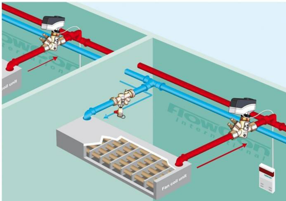
Система тепло-/холодоснабжения
