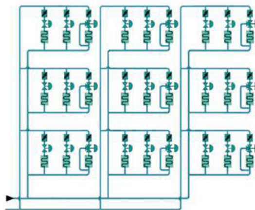
Динамические балансировочные клапаны
